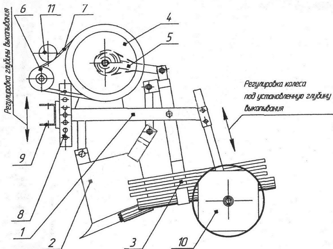
Рис.1. Общий вид картофелекопалки (на примере модели КМ1080).
