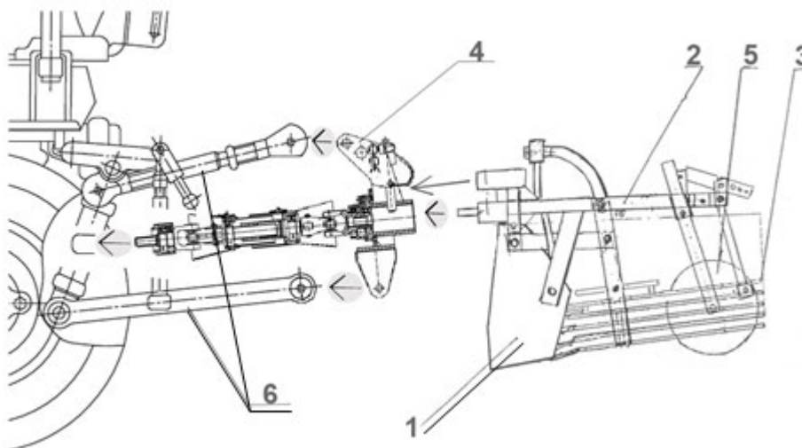
Рис.1. Общий вид картофелекопалки.
