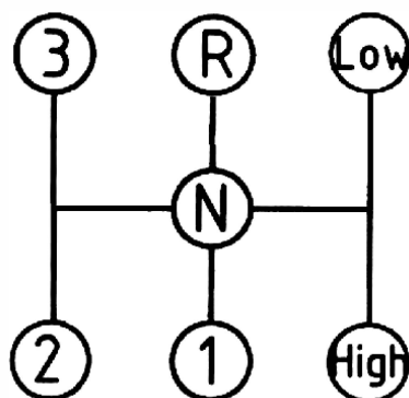
Рис. 2. Схема переключения передач КПП типа (3 вперед + 1 назад) x2.
