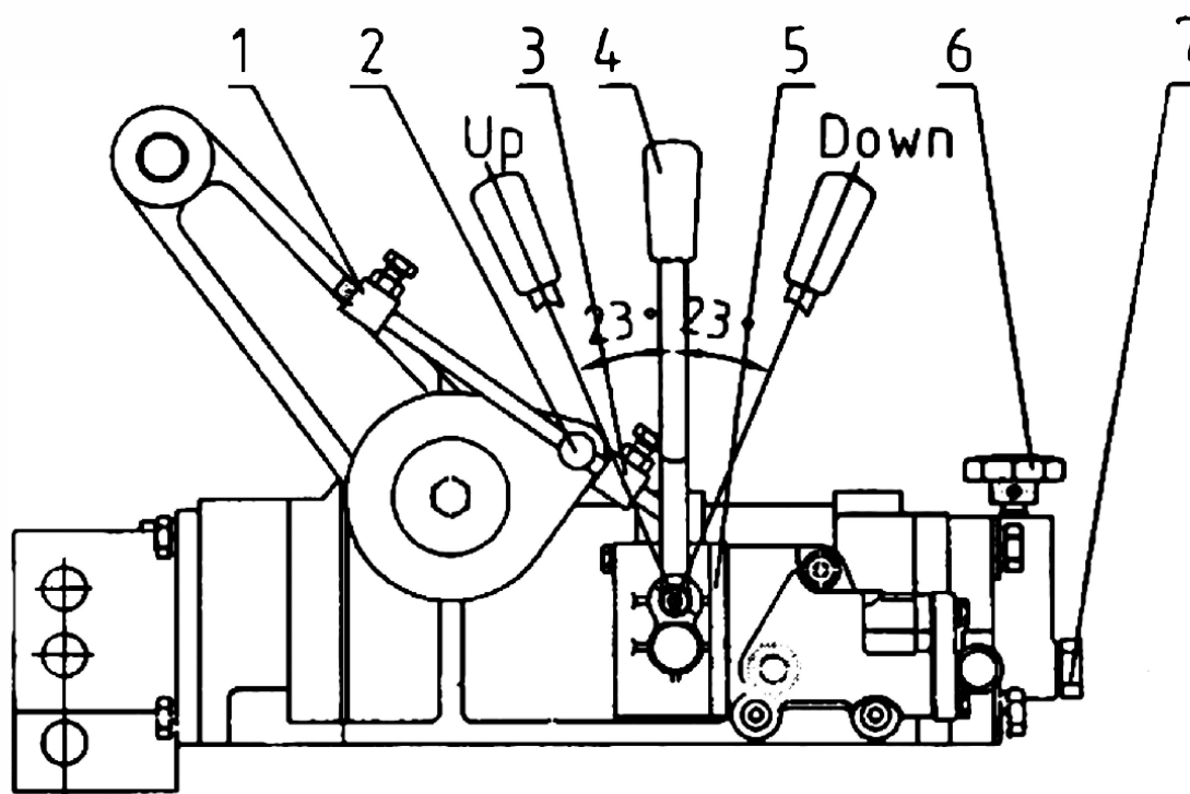
Рис. 16. Гидравлический подъемник.
