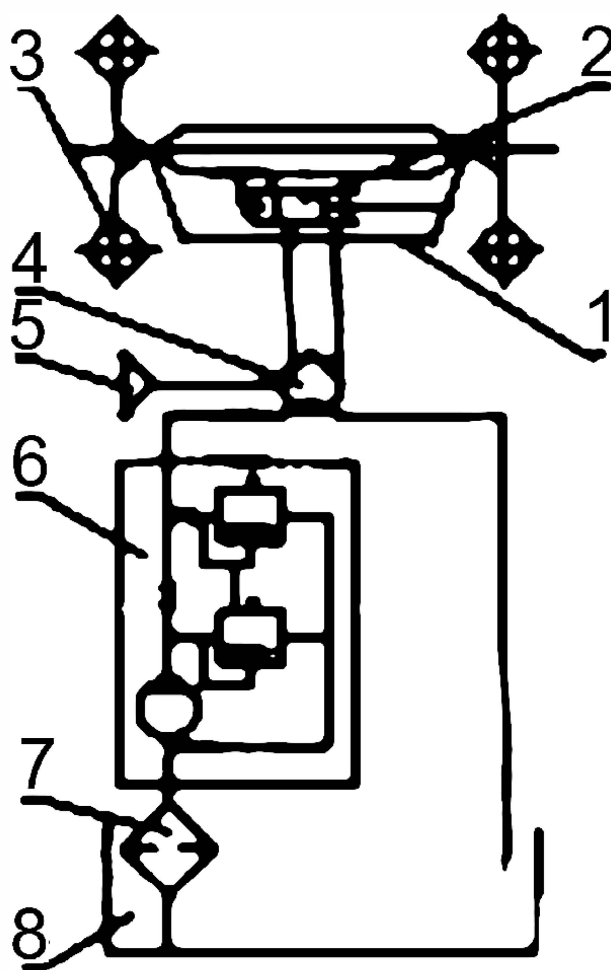
Рис. 10. Принцип действия гидравлического рулевого механизма.
